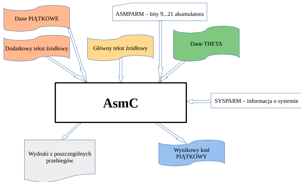
Konfiguracja wejścia/wyjścia assemblera
